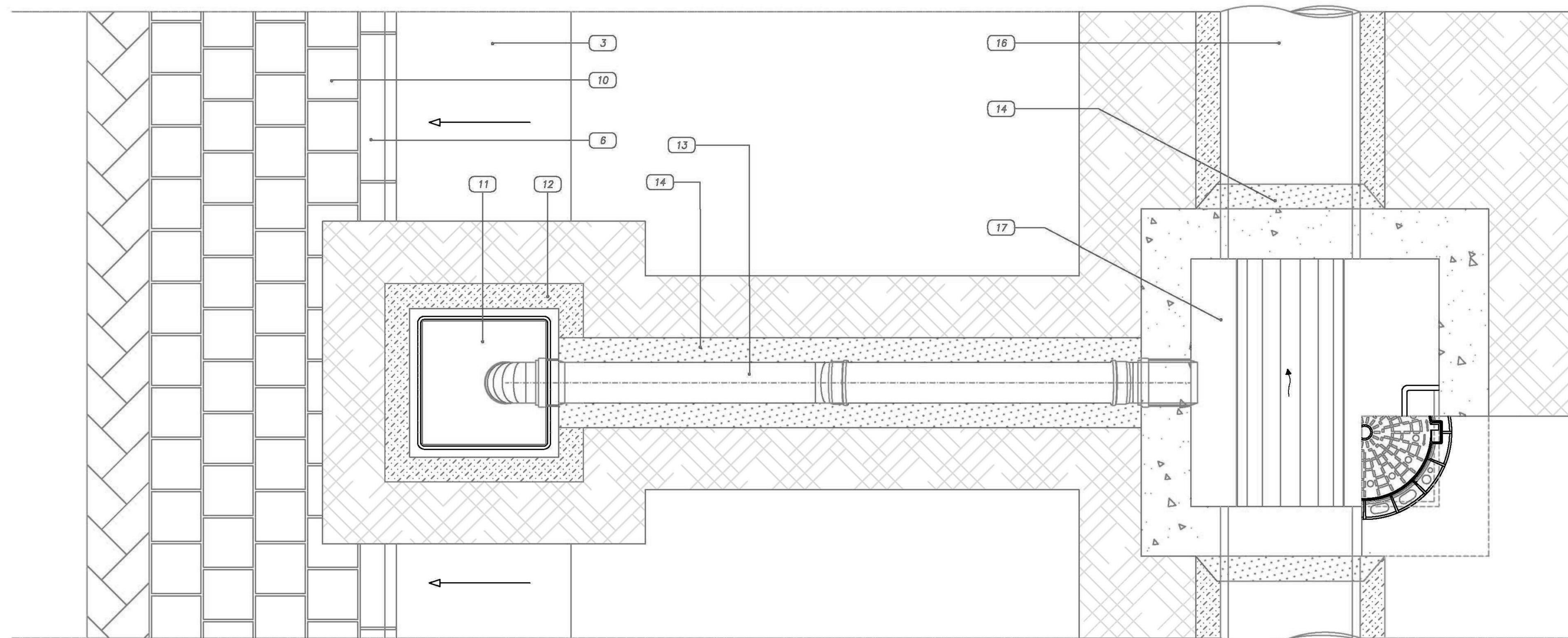
COLLEGAMENTO CADITOIA - POZZETTO A TRE VIE VISTA IN PIANTA Scala 1:10
