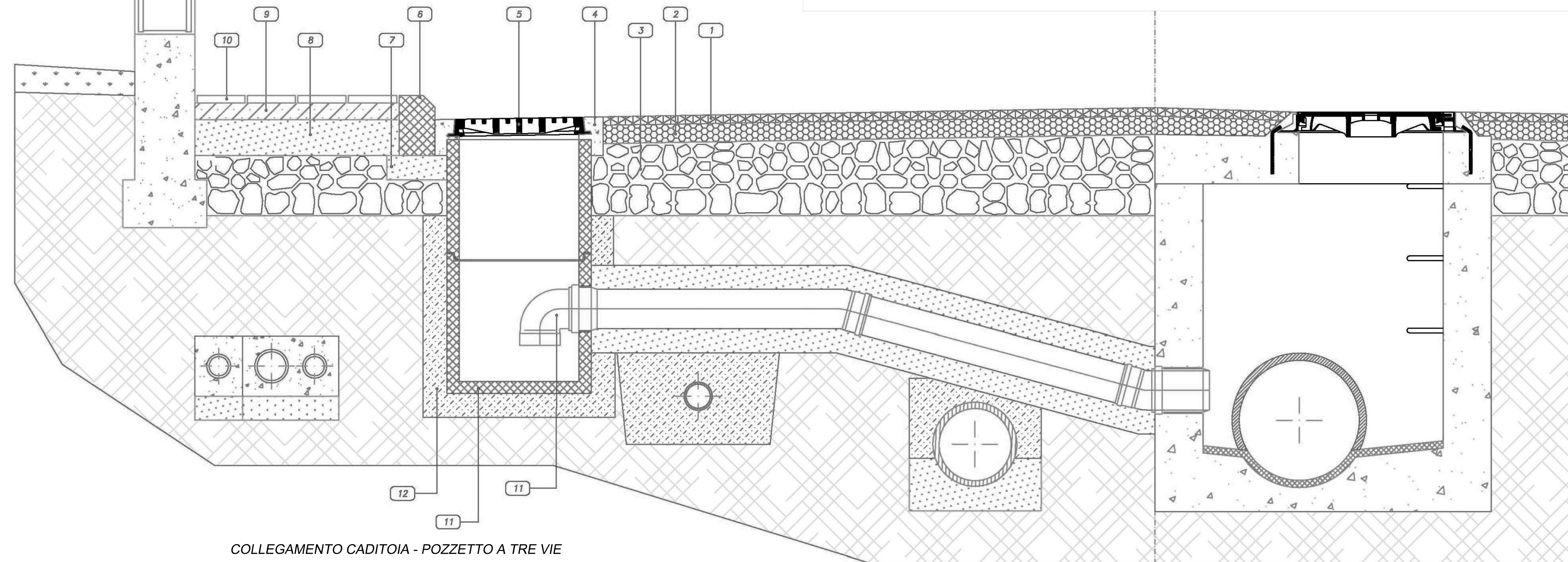
Collegamento caditoia - pozzetto a tre vie Condotta di collegamento: PVC Ø 160 Condotta fognaria: CEMENTO Ø 1000
